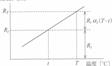
図 10.1 温度による抵抗値の変化
