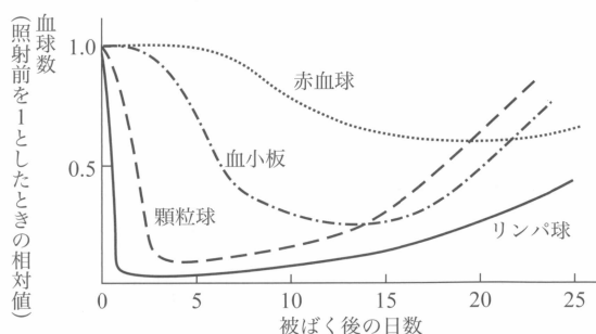
図8.4 放射線照射後の末梢血液中の血球数の変化
