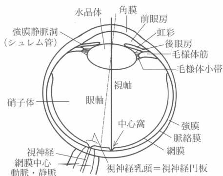
図 7.116 眼球構造
