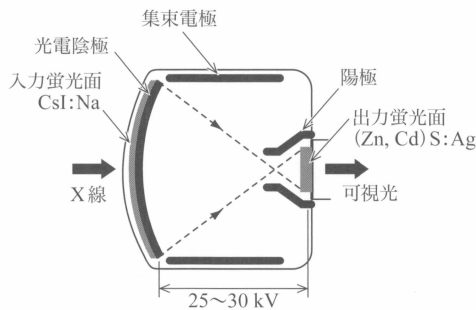
図2.10 イメージインテンシファイアの構造
